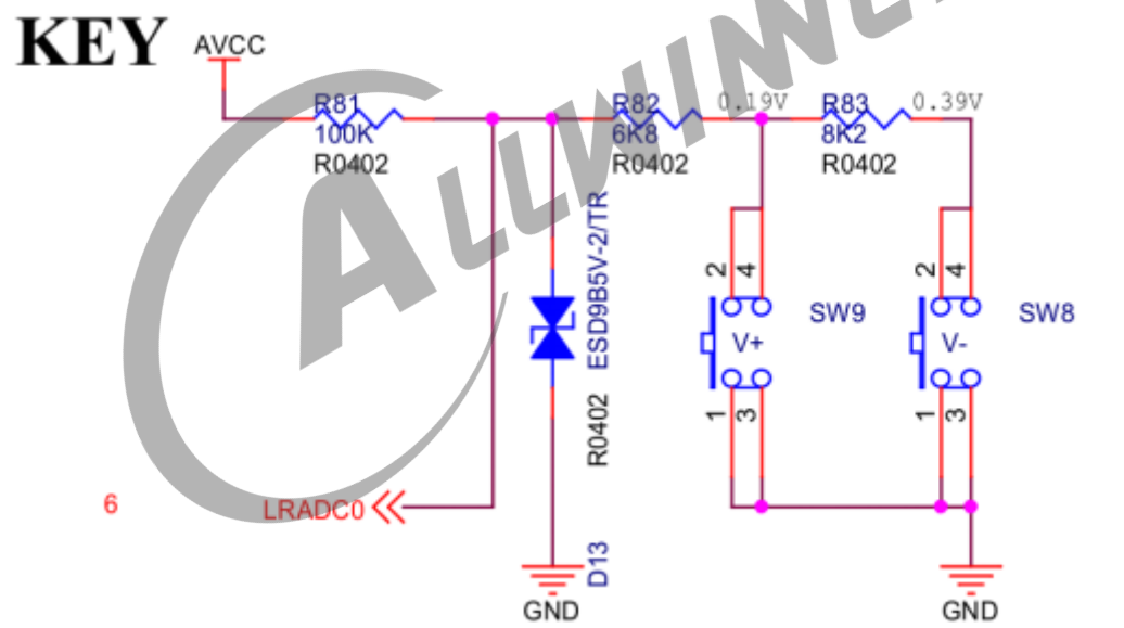
图 4-1: LRADC 按键原理图
